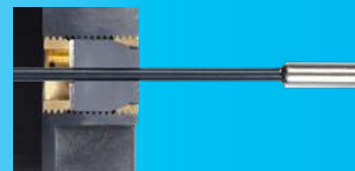
С двумя гайками M20 и принадлежностями для ввода кабеля датчика температуры
