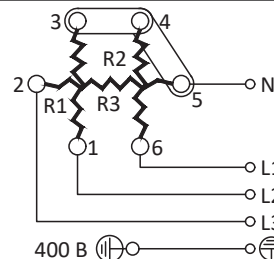
Положение ремней в 3-х фазной сети 380-400 В
