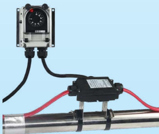
Пример монтажа на двух кабелях теплофикации, с соединительной коробкой Y26 с подъемным кронштейном из нержавеющей стали, для защиты труб от замерзания.
